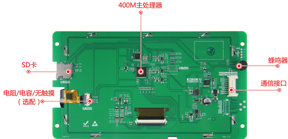
图 1-4 硬件配置图
